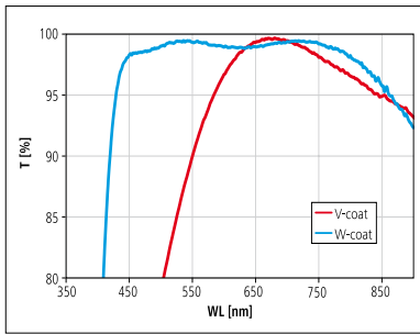
Beispielkurve Antireflexbeschichtungen
